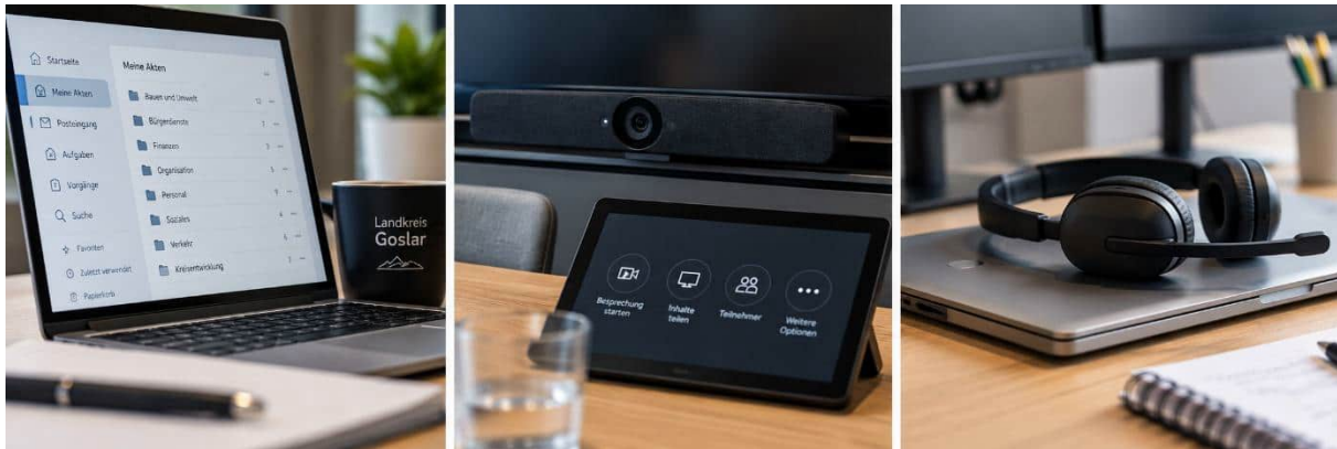
Abbildung 1: Quelle ChatGPT
